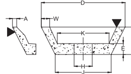
16. Cones Grinding
